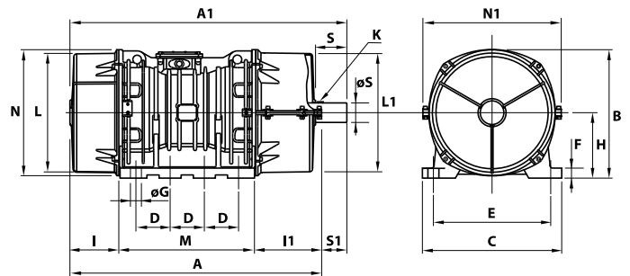
Caractéristiques dimensionnelles (mm)
