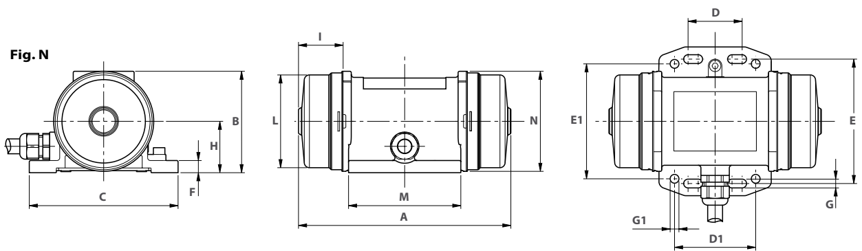
Caractéristiques dimensionnelles (mm)
