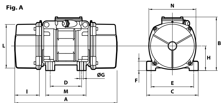
Caractéristiques dimensionnelles (mm)
